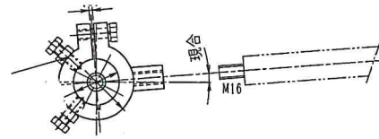
A部詳細
